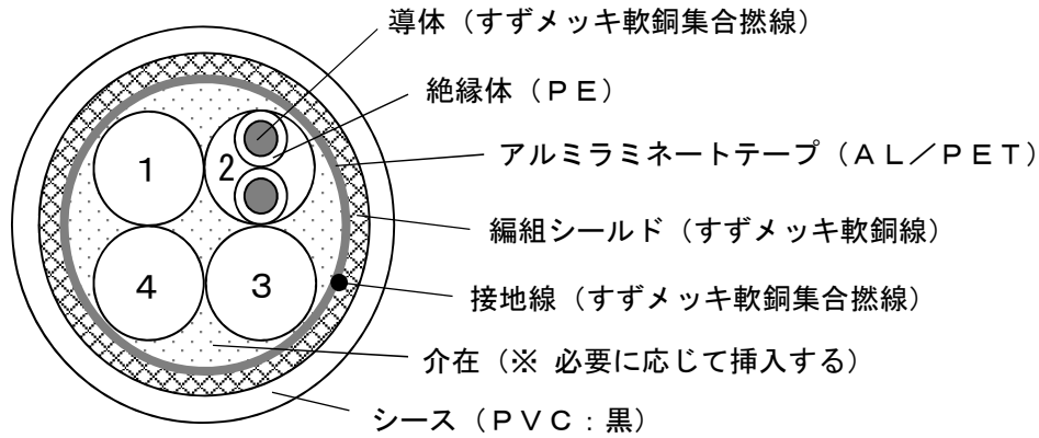
付図 - 1 (断面図)
